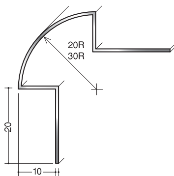
丸面出隅20-10 (DR-920) 丸面出隅30-10 (DR-930)
