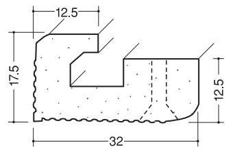
コーナーベース12.5 2.6m/30本入/ビス穴φ3.3/ピッチ200mm
