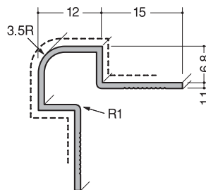
6-3.5R Gホワイト 2.73m
