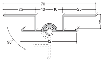
●フリー入隅2型
