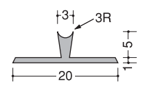
6T型(目地) シルバーのみ 2.73m
