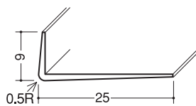
GLコーナー9×25 クリーム／2.5m／100本入 2.73m／100本入(取寄品) ※テープ付もごさいます。
