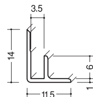
入隅スーパー3 白 2.5m/150本入 2.73m/150本入(取寄品)
