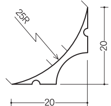
階段コーナー25R グレー/1.82m/50本入
