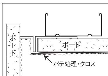
クロス見切Z-906 白/1.82m/100本入
