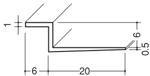
クロス見切Z-606 白/1.82m/150本入
