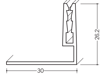
塩ビGW・L型ベースBK-25型
