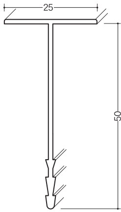
塩ビGW・T型カバーKT-50型
