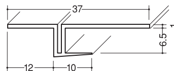
クロス見切6型 白/2.3m/150本入
