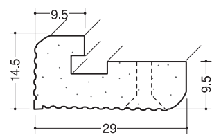
コーナーベース9.5 2.6m/40本入/ビス穴φ3.3/ピッチ200mm
