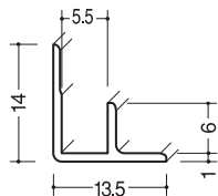
入隅スーパー5 120本入
