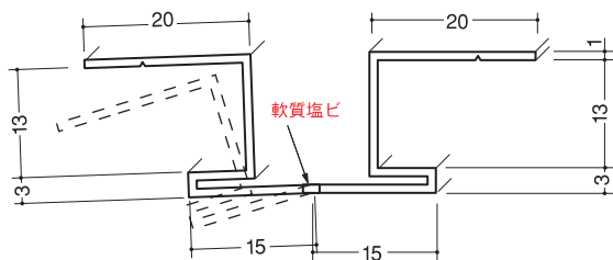
フリーズジョイナー12 白/2.5m/40本入
