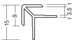
出隅用 (C形状)
