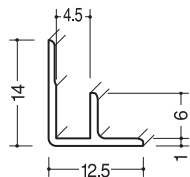
入隅スーパー4 120本入
