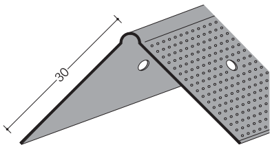
亜鉛コーナービート 2.43m/50本入/t=0.4
