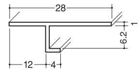
クロス見切縁TVC-6 200本入
