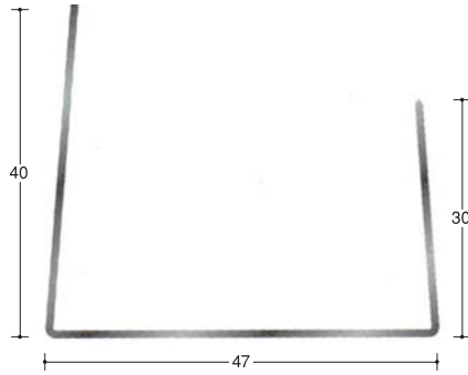
ランナー45 3m・6本束
