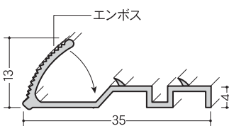
アルミコーナーグリップB DSタイプ/3.64m
