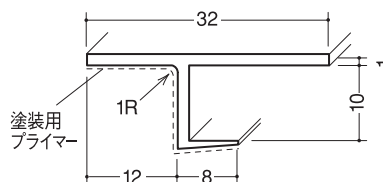
ペンキ見切PPZ-9
