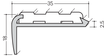
アルミノンスリップALY-135
