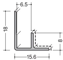
6.5FB Gホワイト 2.73m
