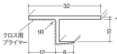
クロス見切CP-9
