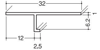
クロス見切縁T-6 150本入
