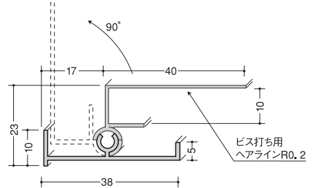
●フリー廻り縁
