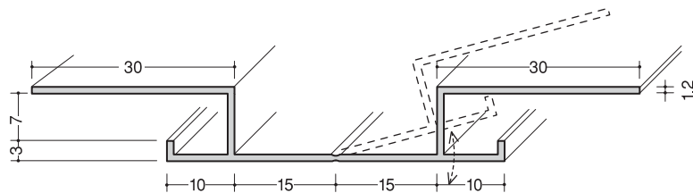
アルミフリーズジョイナー6
