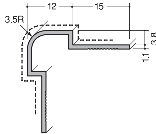
3-3.5R Gホワイト 2.73m
