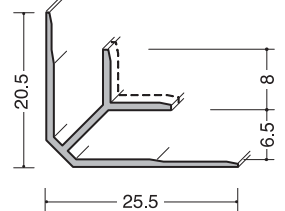
6.5BC Gホワイト 2.73m
