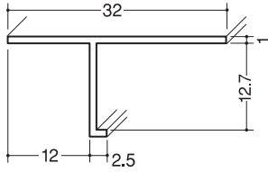
クロス見切縁T-12 100本入
