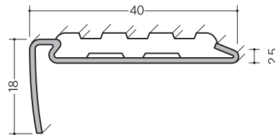
ステンノンスリップSTY-140
