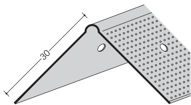
アルミコーナービート 2.43m/50本入/t=0.4
