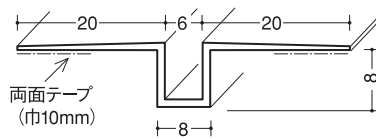
ハット目地6テープ付 40本入
