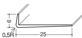
GLコーナー6×25 クリーム／2.5m／100本入 2.73m／100本入(取寄品) ※テープ付もごさいます。
