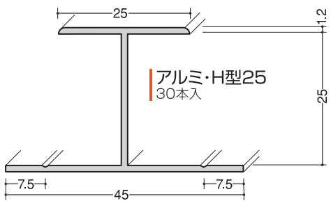
アルミ H型 色：シルバー 長さ：2.73m
