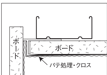
クロス見切Z-606 白/1.82m/150本入
