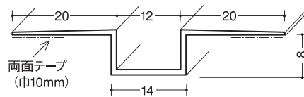
ハット目地12テープ付 40本入
