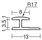
平目地用 (A形状)
