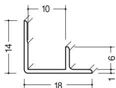
入隅スーパー9 80本入
