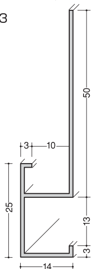
DX-129 (D型16) 3m, 30本入
