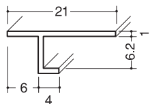
クロス見切縁TV-606 200本入
