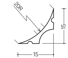
階段コーナー20R グレー/1.82m/50本入
