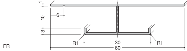
●オールアルミジョイント 3m
