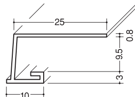
A3-9.5 (岩綿板用)
