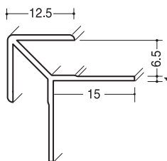
GKA-6.5 Gホワイト 2.73m/50本入
