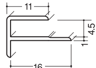
出隅スーパー4.5 120本入
