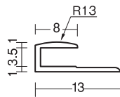
見切り用 (B形状)
