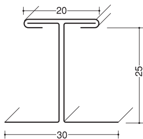
カラー鉄板H型25 クリーム／受注品
