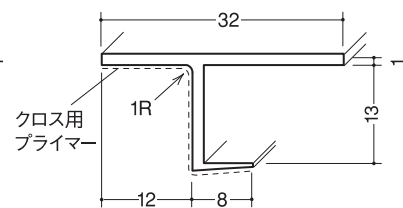
クロス見切CP-12
