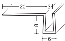
MB目地3 100本入
