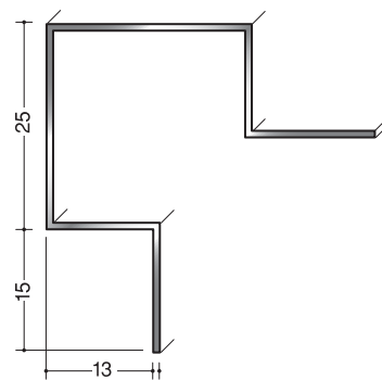
ステン角型出隅12
