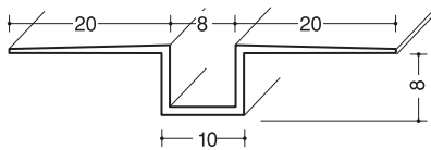
ハット目地8 40本入
