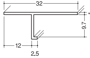
クロス見切縁T-9 100本入
