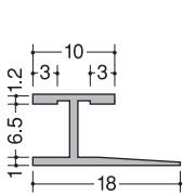
6SH型(目地) 2.43m 2.73m 1A・2B・3B
