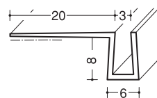
MB目地3テープ付 100本入
