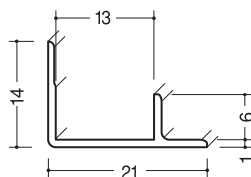
入隅スーパー12 80本入
