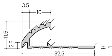
アルミパンチボーダー 3.64m
