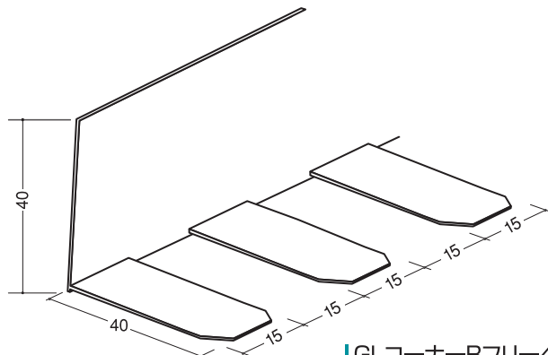
GLコーナーRフリー40 100本入
