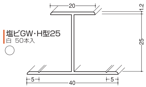
塩ビ H型 色：白 長さ：2.73m
