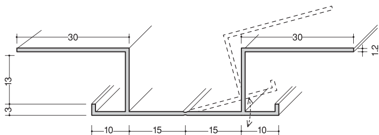
アルミフリーズジョイナー12
