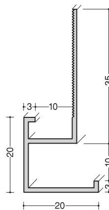
DX-99 3m, 30本入
