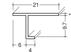
クロス見切縁TV-609 150本入
