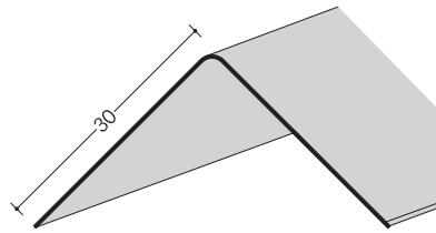
アルミ折コーナー 2.73m/t=0.35
