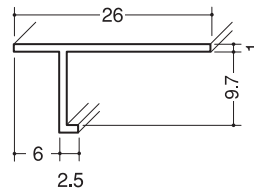
クロス見切縁T-609 150本入
