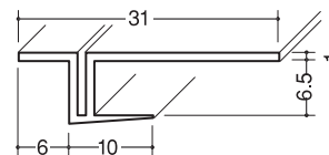
クロス見切FP-6 白/1.82m/100本入
