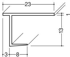
クロス見切12型 白/2.3m/100本入
