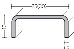
ステンフロアー目地 25mm/4m 30mm/4m
