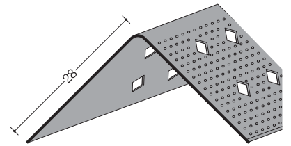
亜鉛かどだしコーナー 2.73m/50本入/t=0.4
