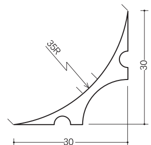
階段コーナー35R グレー/1.82m/50本入
