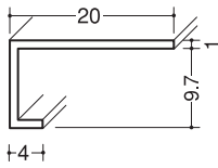
クロス見切TC-9 100本入
