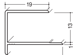
出隅スーパー12.5 50本入
