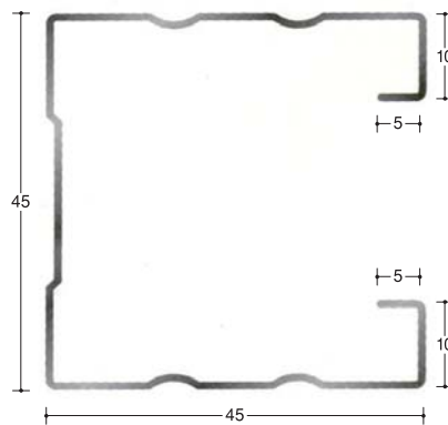
スタット45 3m・10本束
