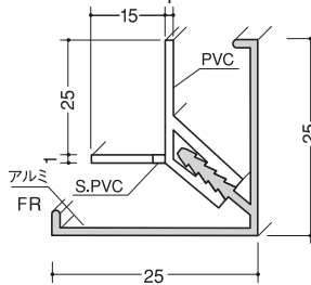
●フリー入隅2型
