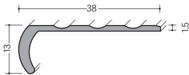
真鍮ノンスリップBY-38
