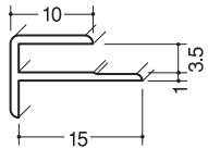
出隅スーパー3.5 120本入
