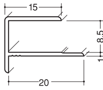
出隅スーパー8.5 70本入
