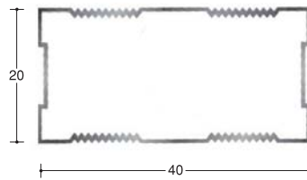
角スタット2040 3m・6本束
