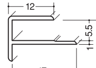
出隅スーパー5.5 100本入
