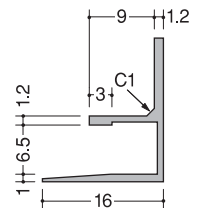
6SL型(入隅) 2.73m
