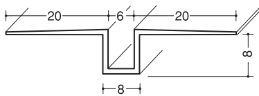
ハット目地6 40本入
