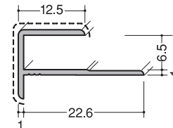
6.5FA Gホワイト 2.73m
