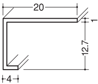
クロス見切TC-12 100本入
