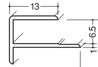
出隅スーパー6.5 100本入
