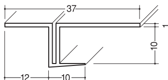
クロス見切FP-9 白/1.82m/100本入
