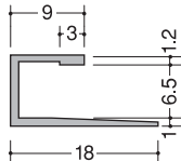
6SU型(仕舞) 2.43m 2.73m 1A・2B・3B
