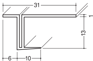
クロス見切FPC-12 白/1.82m/100本入
