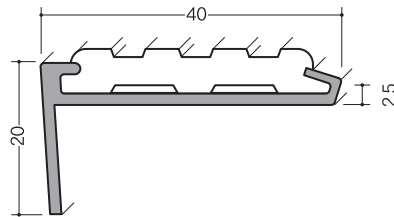
真鍮ノンスリップBY-140
