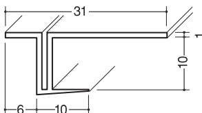
クロス見切FPC-9 白/1.82m/100本入
