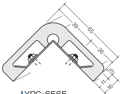
YPC-6565 ビニール製/1m・2m
