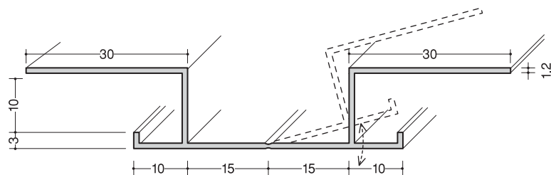
アルミフリーズジョイナー9
