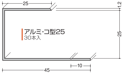
アルミ コ型 色：シルバー 長さ：3m
