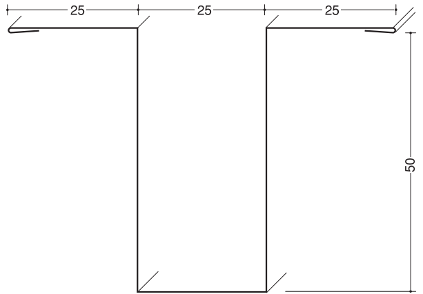
カラー鉄板ハット50 クリーム／受注品
