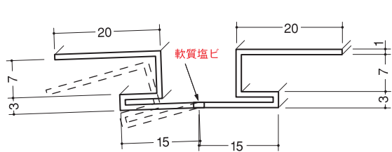
フリーズジョイナー7 白/2.5m/50本入
