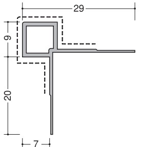
シブ出隅I型 Gホワイト 2.73m
