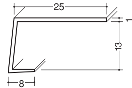
クロス見切AP-12 150本入
