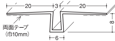
ハット目地3テープ付 100本入
