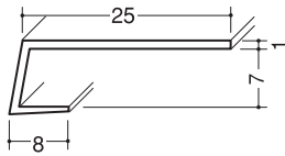
クロス見切AP-6 150本入
