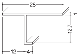
クロス見切縁TVC-12 100本入
