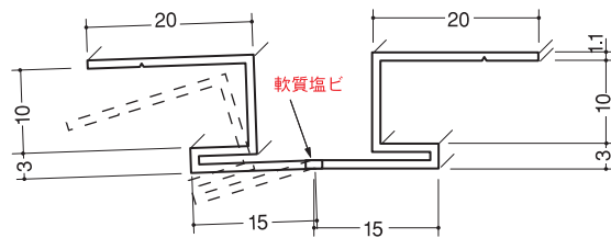
フリーズジョイナー9 白/2.5m/50本入
