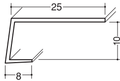
クロス見切AP-9 150本入
