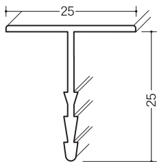
塩ビGW・T型カバーKT-25型
