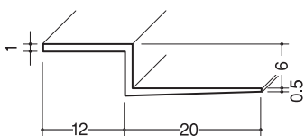
クロス見切FPC-12 白/1.82m/100本入
