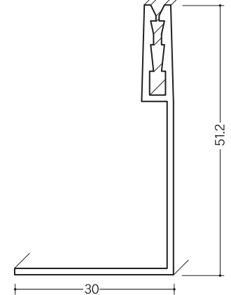
塩ビGW・L型ベースBK-50型
