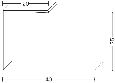
カラー鉄板コ型25 クリーム・グレー・黒／グレー・黒は受注品
