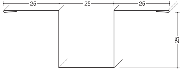
カラー鉄板ハット25 クリーム／受注品
