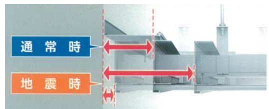
図は壁際クリアランス(C寸法)100mm
