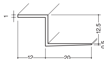
クロス見切Z-1212 白/1.82m/100本入
