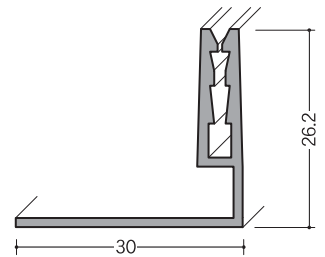
塩ビ・L型ベースBK-25型 グレー／60本入
