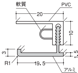
●アルミ廻り縁(ベース:樹脂製)
