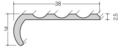
アルミノンスリップALY-38
