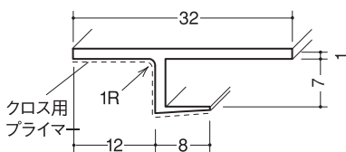
クロス見切CP-6
