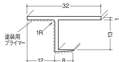
ペンキ見切PPZ-12
