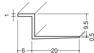
クロス見切Z-906 白/1.82m/100本入
