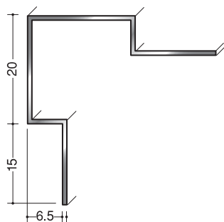
ステン角型出隅6
