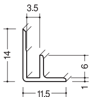
入隅スーパー3 150本入
