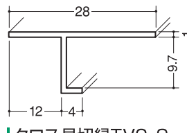
クロス見切縁TVC-9 100本入
