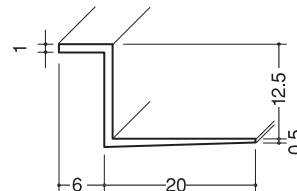
クロス見切Z-1206 白/1.82m/100本入
