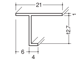
クロス見切縁TV-612 150本入
