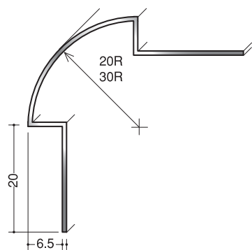
丸面出隅20-6.5 (DR-620) 丸面出隅30-6.5 (DR-630)
