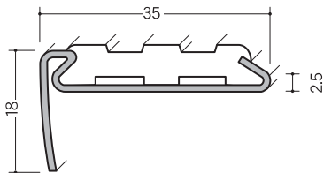
ステンノンスリップSTY-135
