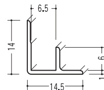
入隅スーパー6 120本入
