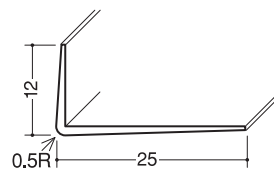
GLコーナー12×25 クリーム／2.5m／100本入 2.73m／100本入(取寄品) ※テープ付もごさいます。
