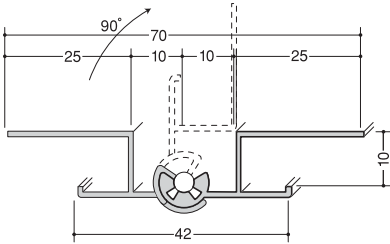
●フリー出隅2型
