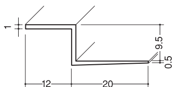
クロス見切Z-912 白/1.82m/100本入
