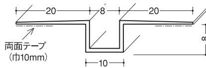
ハット目地8テープ付 40本入
