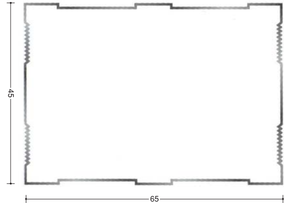
角スタット4565 3m・4本束
