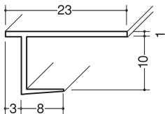
クロス見切9型 白/2.3m/200本入
