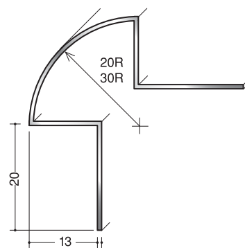
丸面出隅20-13 (DR-1220) 丸面出隅30-13 (DR-1230)
