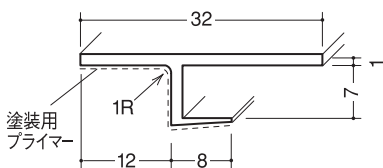
ペンキ見切PPZ-6
