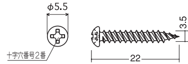
ハット型用小頭ビス 3.5×22 200本入/袋(ユニクロ/ホワイト/ブラック) 1000本入/小箱(ユニクロ)
