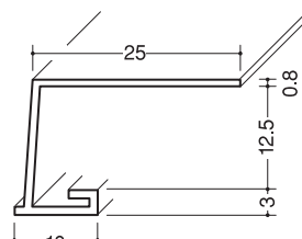
A3-12.5 (岩綿板用)
