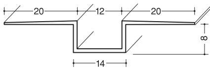
ハット目地12 40本入
