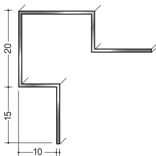
ステン角型出隅9
