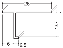
クロス見切縁T-612 150本入
