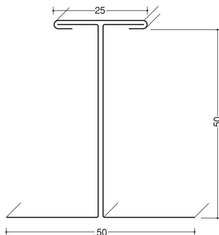
カラー鉄板H型50 クリーム／受注品
