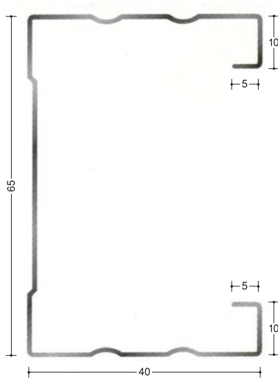
スタット65 3m・6本束
