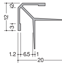
6SA型(出隅) 2.73m
