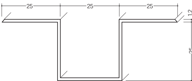
塩ビGW・ハット25型
