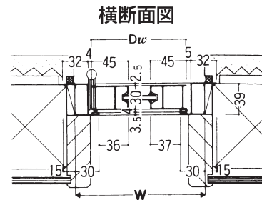
● 把手出寸法表(中框からの出寸法です) 単位:mm
