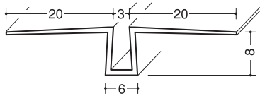
ハット目地3 100本入
