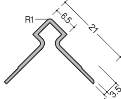
出隅 (Q形状)
