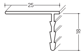
塩ビGW・L型カバーKK-255型
