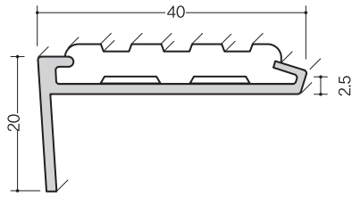
アルミノンスリップALY-140
