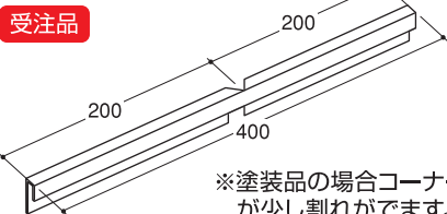
6.5コC、 565コC、 GKC6.5
