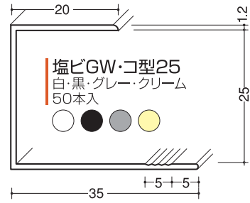
塩ビ コ型 長さ：2.73m
