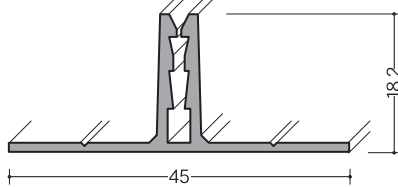
塩ビGW・T型ベースBT型
