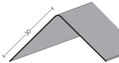
亜鉛折コーナー 2.73m/t=0.4
