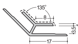
アルミB135°-3.5 2.73m
