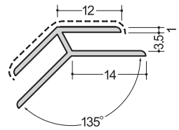
アルミD135°-3 2.73m
