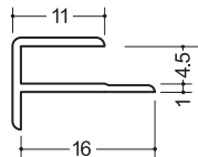
出隅スーパー4.5 2.5m/120本入
