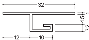
V-4 1.82m/100本入
