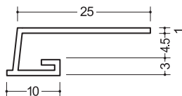
A3-4.5 1.82m/100本入
