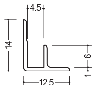
入隅スーパー4 2.5m/120本入
