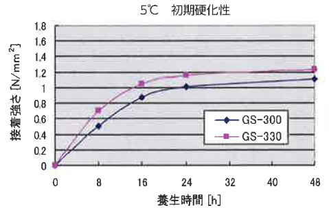
※平面引張強さ (化粧けい酸カルシウム板×フレキ板)
