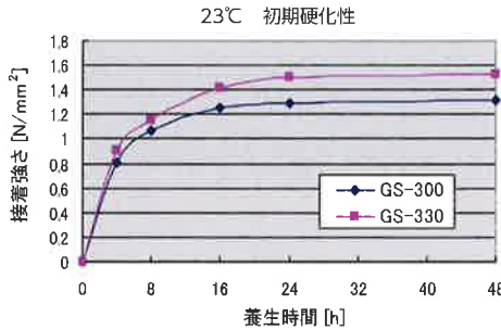
※平面引張強さ (化粧けい酸カルシウム板×フレキ板)
