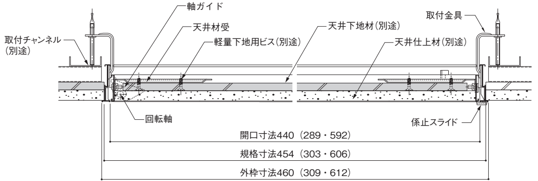
本図は□454を示す。( )内寸法は(□303・□606)を示す。
